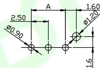
P.C.B LAYOUT(T=1.6mm)
