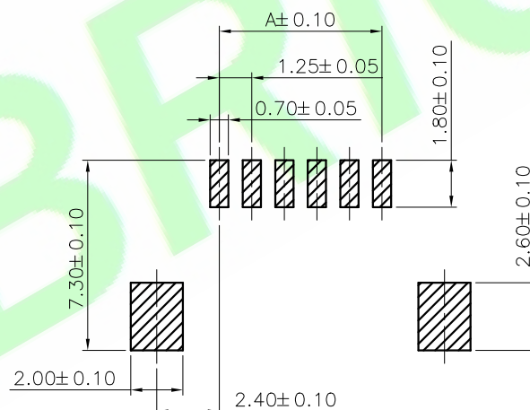
P.C.B. LAYOUT
